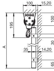
S4110/3 mit Führungsschiene Aluminium avec coulisseaux en aluminium
