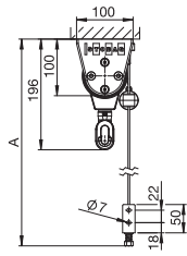
S4110/1 mit Drahtseilführung Inox avec guidage par câbles inox
