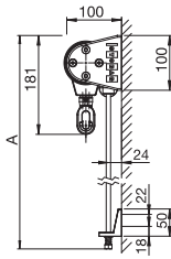
S4110/2 mit Stangenführung Chromstahl avec tiges de guidage en acier chromé
