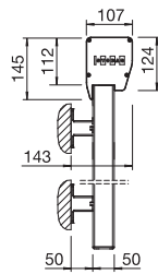
Wandmontage mit eckigem Kasten Montage en façade avec caisson carré
