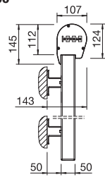
Wandmontage mit rundem Kasten Montage en façade avec caisson arrondi
