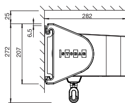
Wandmontage mit eckigem Ausfallprofil Montage en façade avec barre de charge anguleuse
