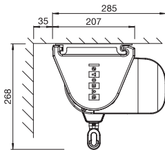
Deckenmontage Ausfallprofil abgerundet Montage sous dalle Barre de charge arrondie
