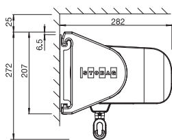
Wandmontage Ausfallprofil abgerundet Montage en façade Barre de charge arrondie
