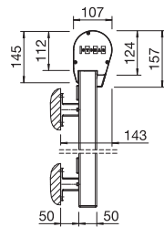
Wandmontage mit rundem Kasten Montage en façade avec caisson arrondi
