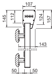
Wandmontage mit eckigem Kasten Montage en façade avec caisson carré
